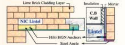
طريقة تثبيت الزاوية المعدنية على العتبة لتحمل طبقة التغطية الجيرية
