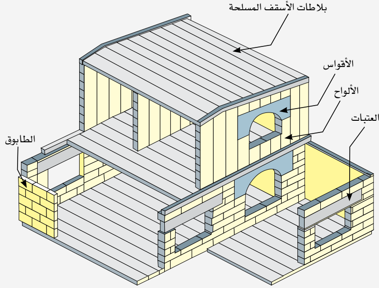
نموذج لاستخدامات الطابوق الأبيض في مختلف أجزاء البناء
