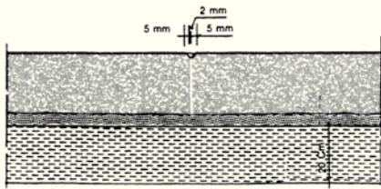
مقطع بلاط مشطوف بدون مونة
