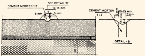
مقطع تركيب بلاط مشطوف بالمونة
