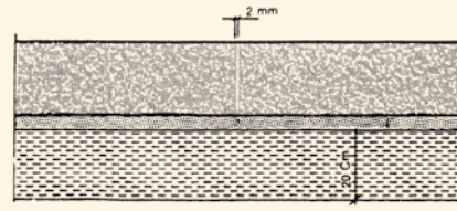
مقطع تركيب بلاط عادي بدون مونة
